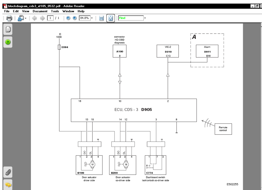
Рис. 6-14 Пример "Блок-схемы"
