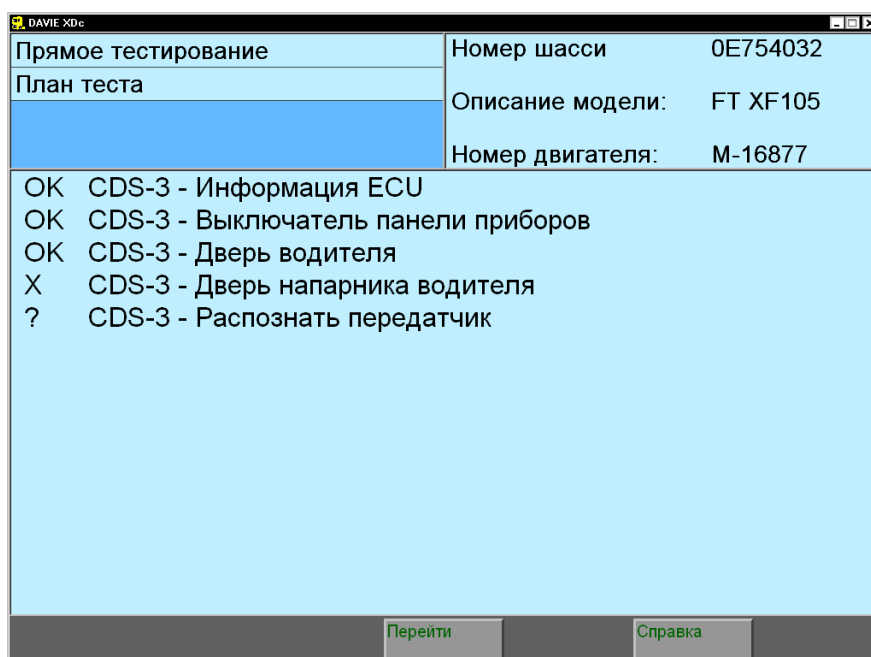
Рис. 6-11 План теста
