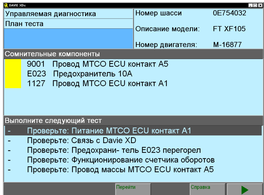
Рис. 7-11 План теста
