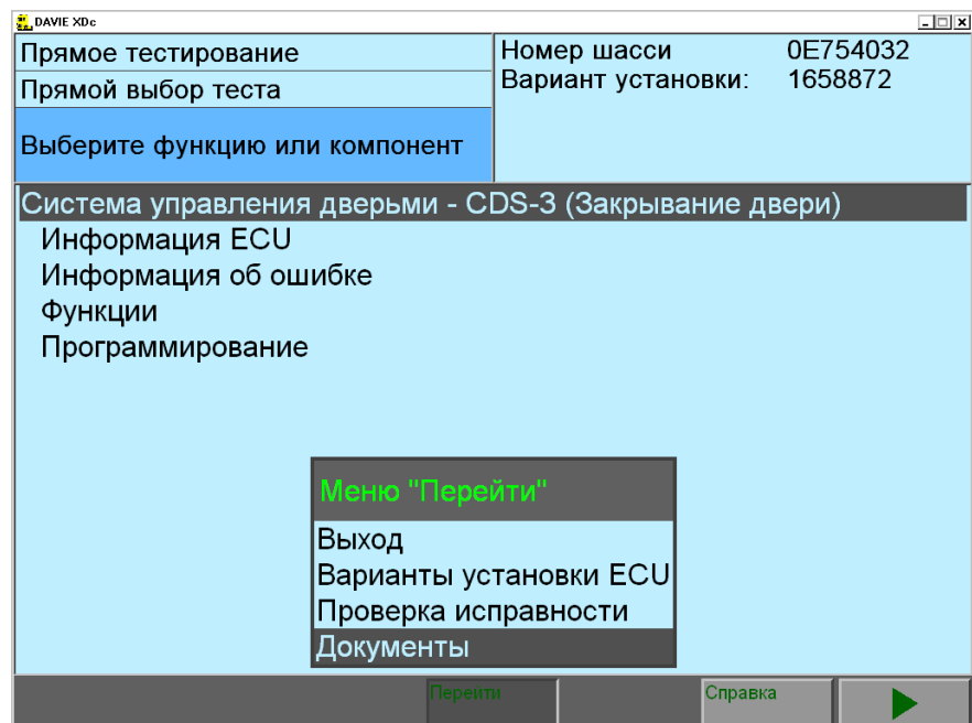
Рис. 6-10 Открытие документов
